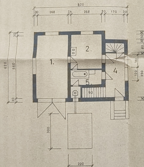
PŘÍZEMÍ
